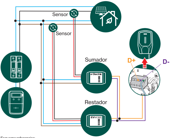
Esquema referencias: 97111 y 97121. Monofásico
