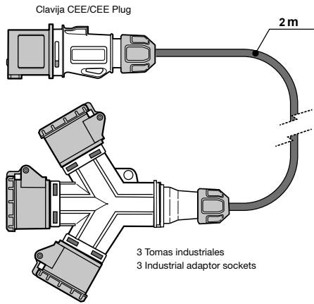
Adaptadores industriales 3 salidas IP54 Industrial adaptors 3 ways IP54
