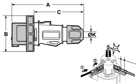
TOP SpeedPRO IP44-54 Base móvil / Mobile socket
