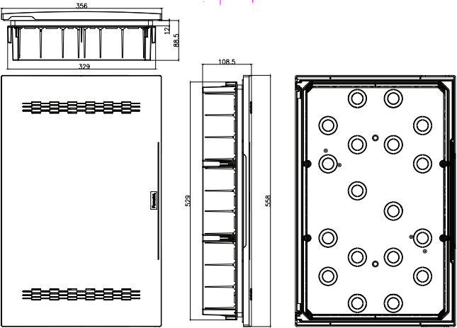
Registro de terminación de red / Network termination register - Ref.Item 32142-F-RE
