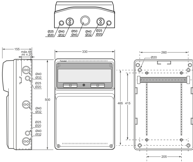
Caja ciega / Blind box - Ref. Item 3977
