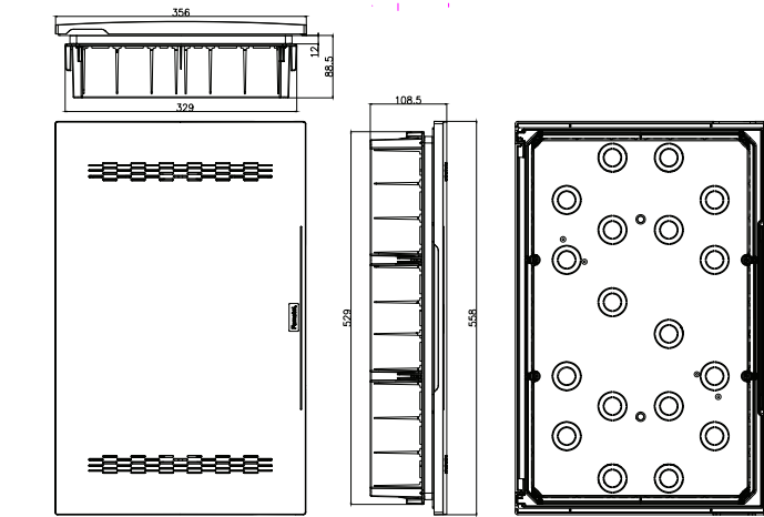
Registro de terminación de red / Network termination register - Ref.Item 32142-RE
