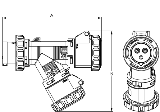
Adaptadores múltiples 2 tomas baja tensión IP67 Multiple adaptors low voltage 50/60 Hz IP67
