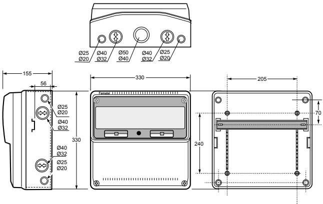
Caja ciega / Blind box - Ref. Item 3952
