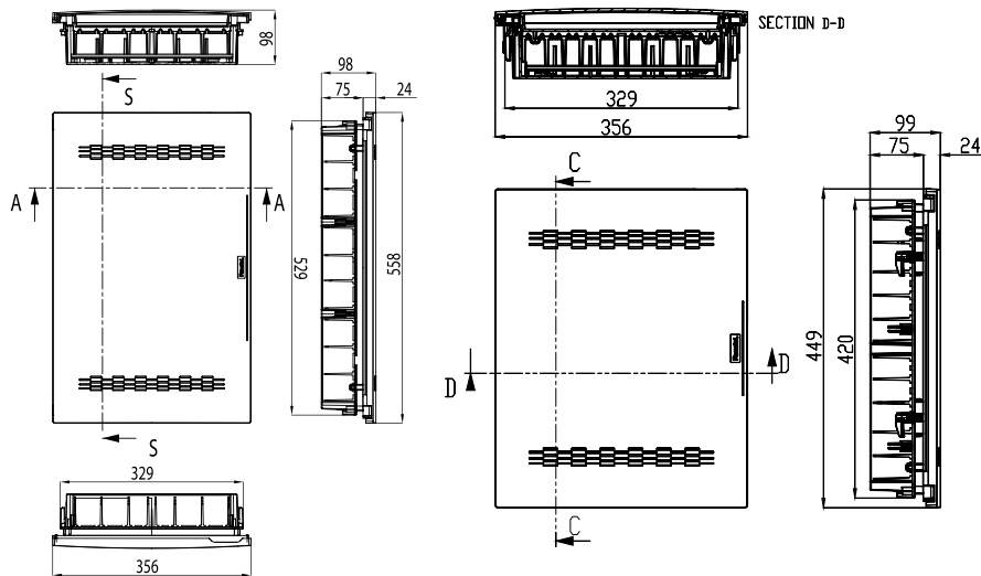
Conjunto de armario y registro de terminación de red / Enclosure and network termination register Set - Ref. Item 32342-F
