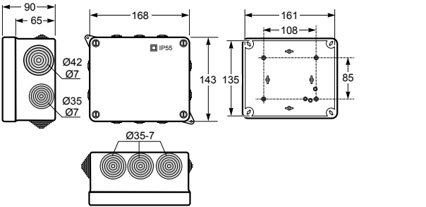
Caja con conos IP55 / Box with cones IP55 - Ref. Item 3014
