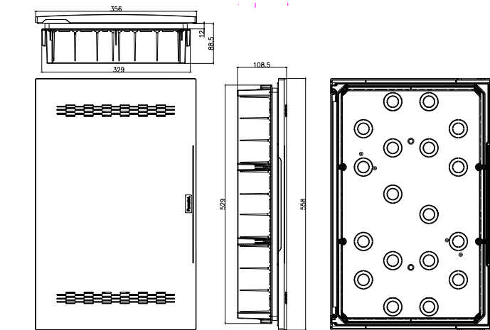
Conjunto 2 registros de terminación de red / 2 Network termination register Set - Ref.Item 32242
