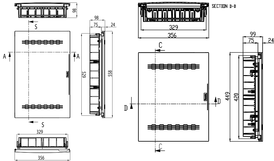
Conjunto 2 registros de terminación de red / 2 Network termination register Set - Ref. Item 32428-F
