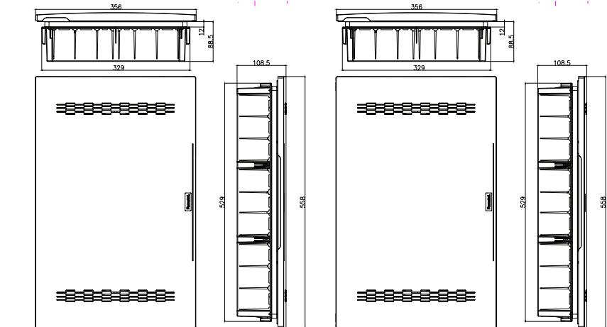
Conjunto de armario y registro de terminación de red / Enclosure and network termination register Set - Ref. Item 32342-F
