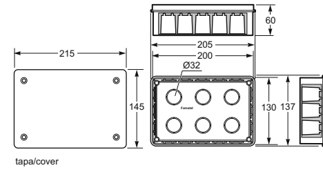
Caja / Box - Ref. Item 3203T
