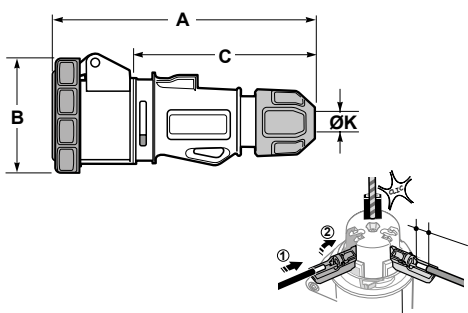
TOP SpeedPRO IP66-IP67 Base móvil / Mobile socket
